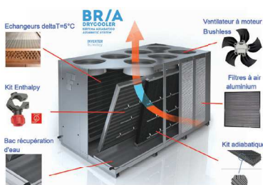
05 Batterie de refroidissement système Adiabatique
