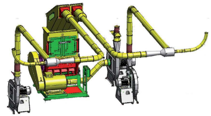
15 Broyage de lisières film
