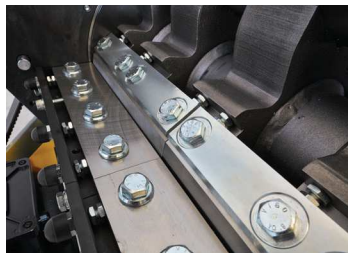
02 Broyeur à couteaux
